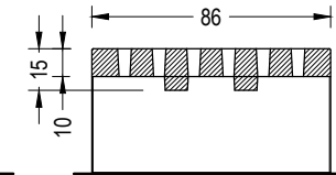
SECCIÓN SECTION
