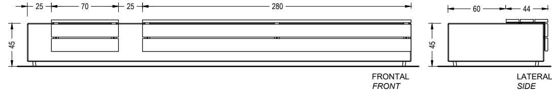
LONGO BANCA + ACCESORIO BANCA + ACCESORIO ASIENTO (2730 kg)
