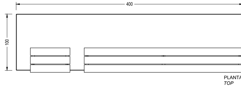
LONGO BANCA LED + ACCESORIO BANCO (2758 kg)
