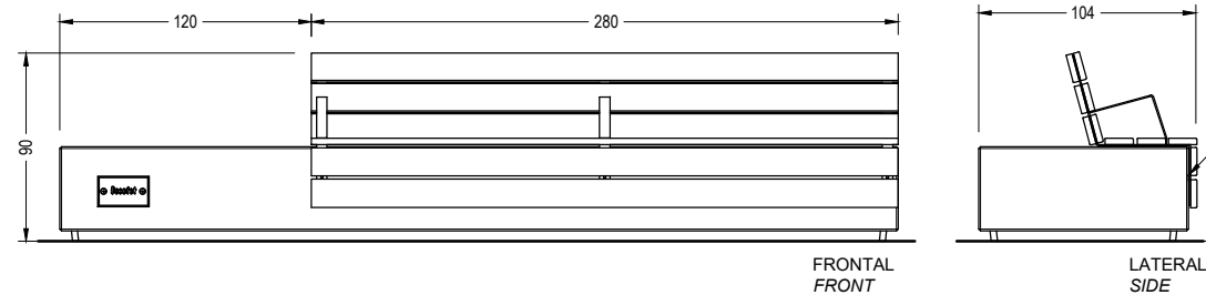
LONGO BANCA LED + ACCESORIO BANCO (2758 kg)
