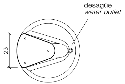
PLANTA INFERIOR
